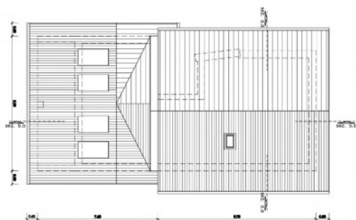
PIANTA COPERTURA
