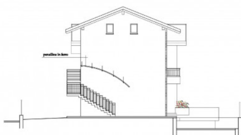
PROSPETTO NORD
