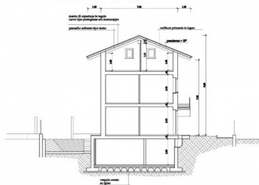
SEZIONE A-A
