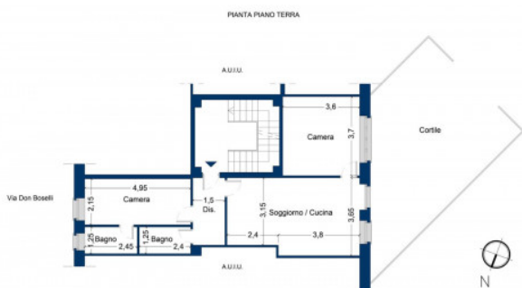
Planimetria unità immobiliare Via Boselli - Alassio
