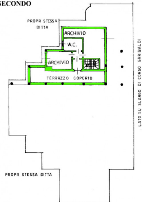
PIANO SECONDO
