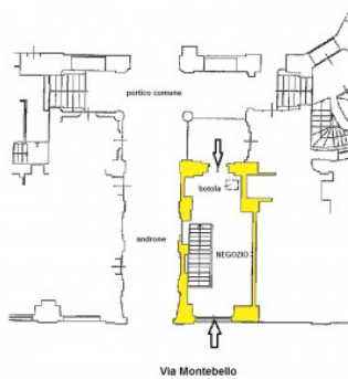
PIANTA PIANO TERRENO (1° f.l.) Hm mt 3,00
