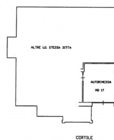
PIANO TERRA (P.T.) H. = 2.07 mt
