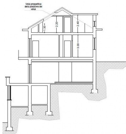
SEZIONE A-A' scala 1/100
