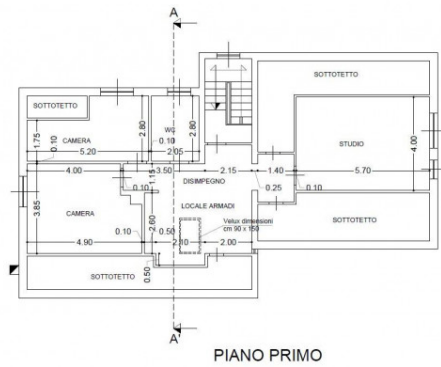
PIANO PRIMO
