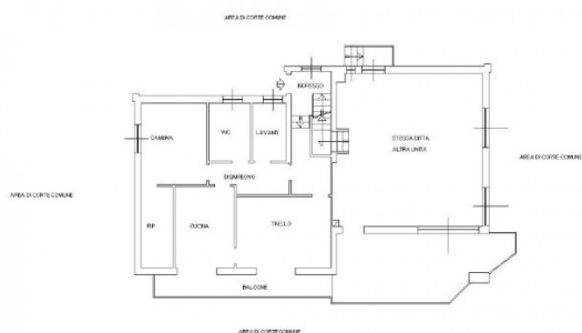
PIANTA PIANO RIALZATO H= 3.00 mt
