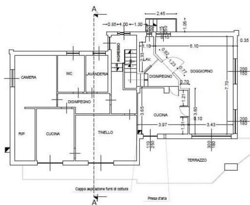
PIANTA PIANO RIALZATO scala 1/100
