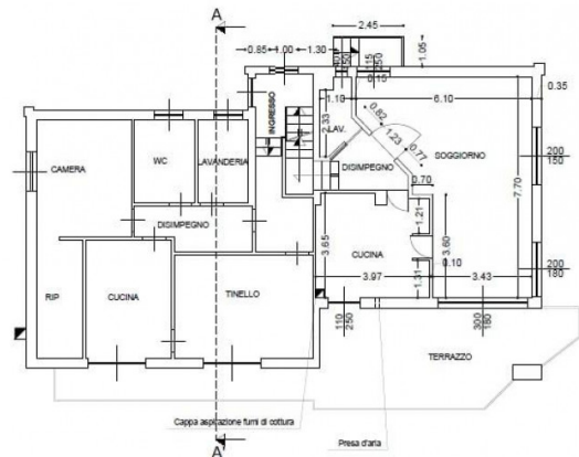
PIANTA PIANO RIALZATO scala 1/100
