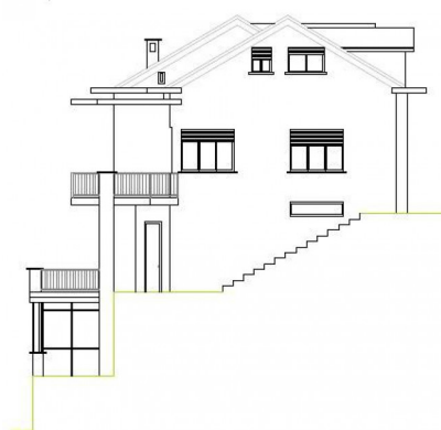
PROSPETTO SUD
