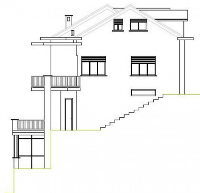
PROSPETTO SUD
