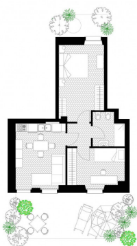
APPARTAMENTO B - piano terra scala 1:50
