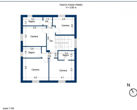
Planimetria unità immobiliare Via Goito 2 - Coniolo (AL)
