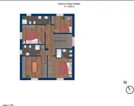
Planimetria unità immobiliare Via Goito 2 - Coniolo (AL)
