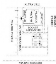
PIANTA PIANO SESTO SOTTOTETTO (7°F.T.)
