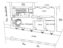
PIANTA PIANO AMMEZZATO altezza mt. 2,50
